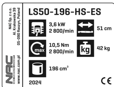
Tabliczka znamionowa
