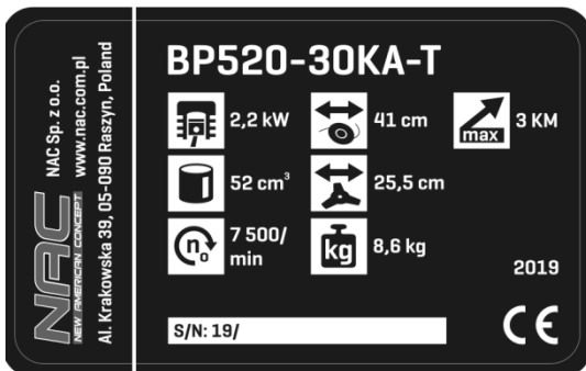
Tabliczka znamionowa
