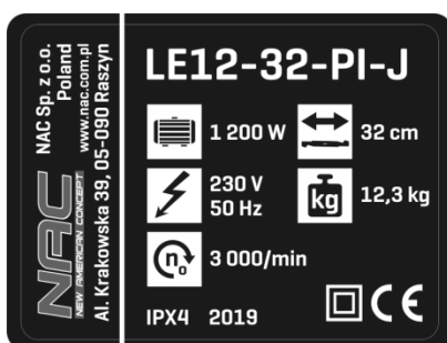
Ttabliczka znamionowa
